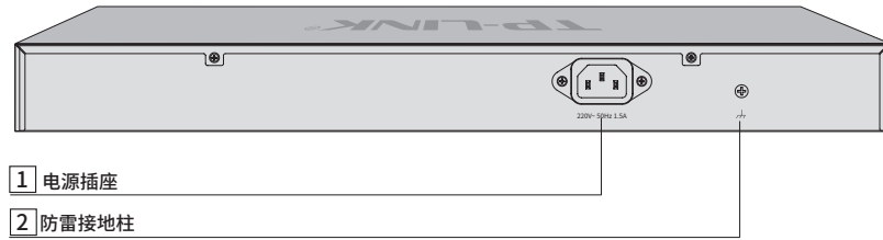
图1-6 TL-SG1218PE后面板示意图
