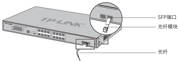
图3-2 SFP端口连接示意图
